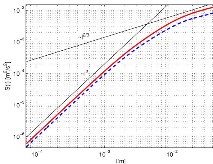
Rys. 5.12: Logarytmiczne wykresy, poprzecznych funkcji struktury z serii nr.1. Przerywana linia – składowa horyzontalna prędkości, ciągła – składowa pionowa.
