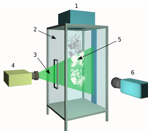
Rys. 4.1: Uproszczony schemat układu eksperymentalnego: 1 - mała komora z generatorem kropelek; 2 - główna komora; 3 - płaszczyna świetlna; 4 - laser; 5 - powietrze chmurowe mieszające się z czystym; 6 - kamera.
